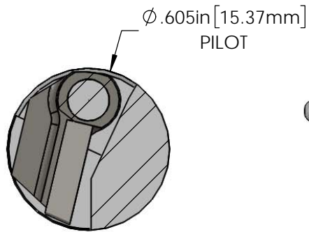
SECTION D-D SCALE 2 : 1
